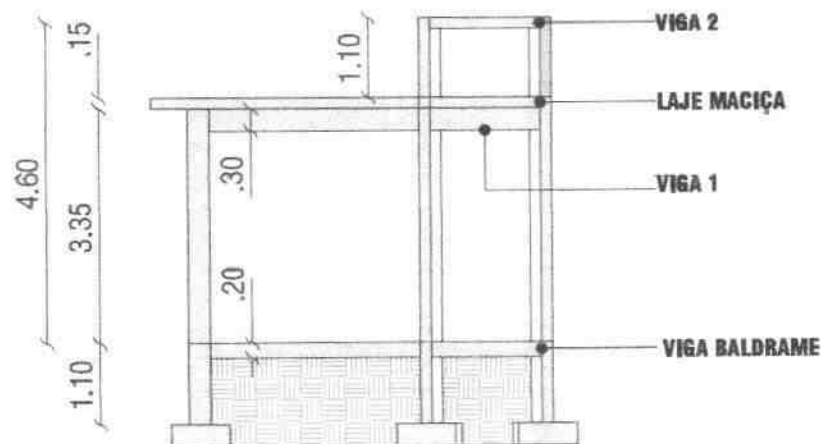
1 CORTE ESTRUTURAL 1:100
