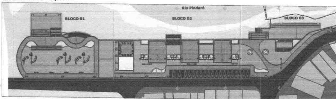
00 PLANTA BAIXA GERAL DA ORLA
