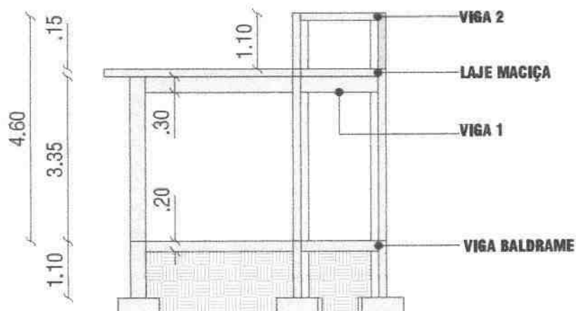
1 CORTE ESTRUTURAL 1:100
