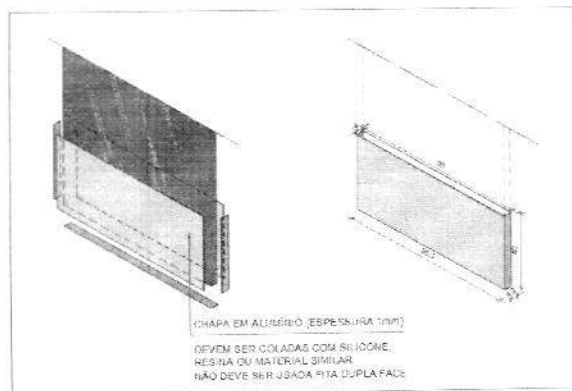
Figura 3 - detalhe chapa metálica para portas de madeira
