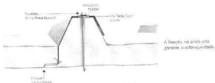
Figura 6 – imagem telha termoacústica
