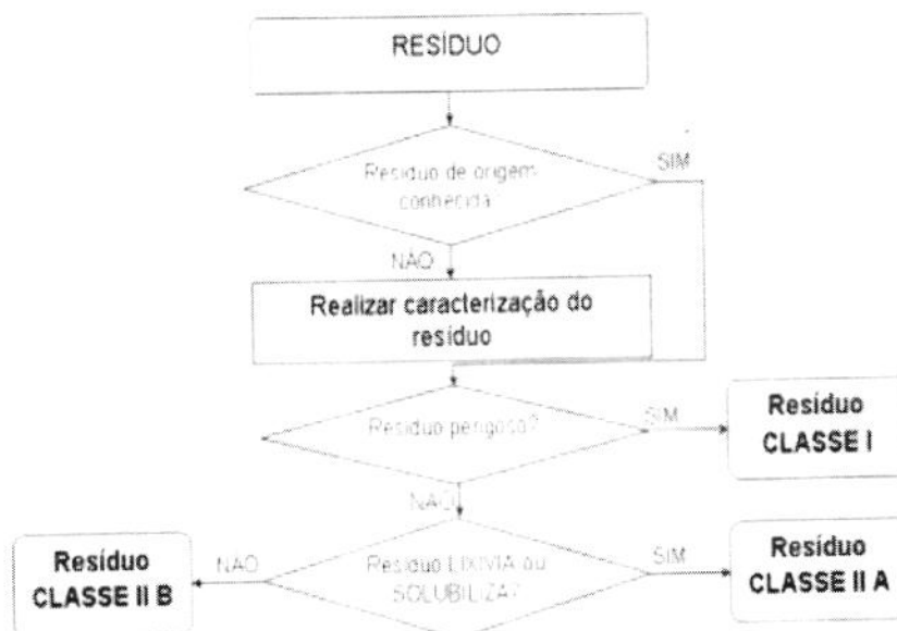
Imagem: Fluxograma de caracterização e classificação dos resíduos sólidos industriais
